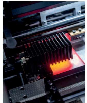
Die Kamera des QualiTronic ColorControl (Bild links) misst jeden Bogen und regelt jeden 10. Bogen. Die ziehmarkenfreie Anlage DriveTronic SIS arbeitet hochpräzise und ist eines der Unique Selling Points der Rapida 76 .
